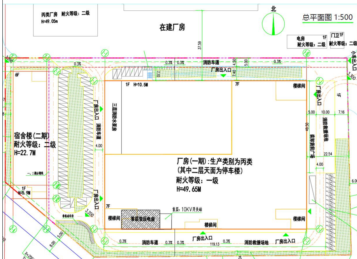
工程总平面布置图
